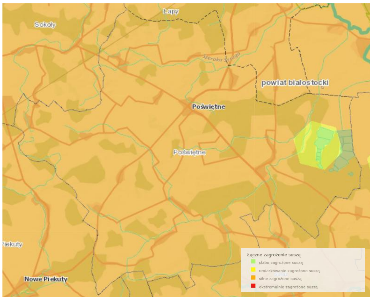
Mapa 31. Mapa prezentująca zagrożenie suszą na terenie gminy Poświętne
