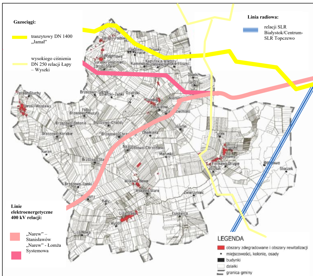
Mapa 21. Model struktury funkcjonalno-przestrzennej – przebieg infrastruktury energetycznej i telekomunikacyjnej na obszarze Gminy Poświętne
