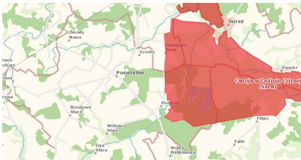
Mapa 7. Obszary chronione na terenie Gminy Poświętne – zasięg przestrzenny
